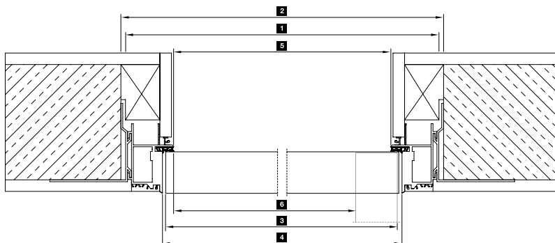
Coupe horizontale avec panneau de porte affleurant
