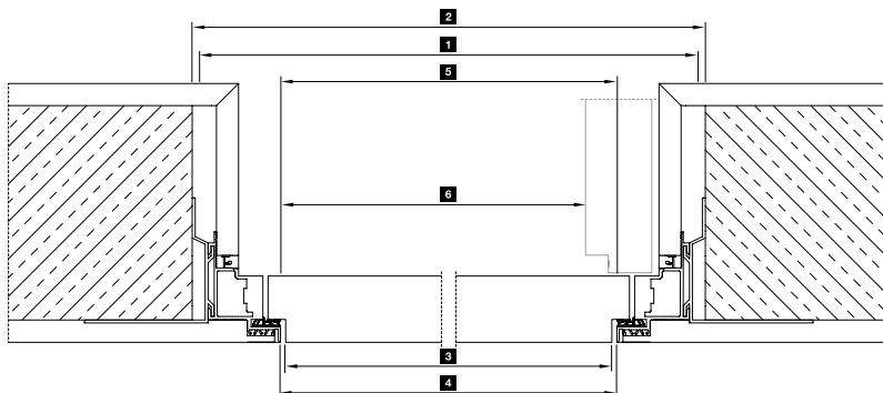
Coupe horizontale avec panneau de porte à ouverture inversée
