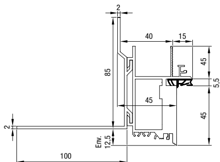
Dimensionnement huissérie de porte Zeroline
